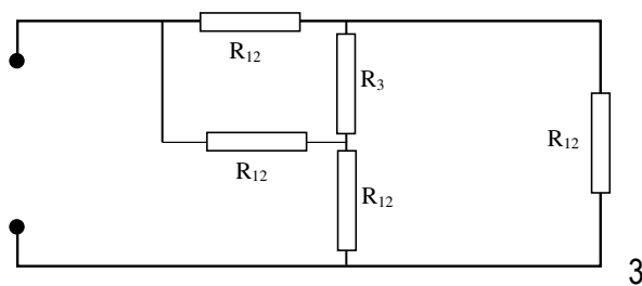
Рис. 2. Эквивалентные схемы подключений
